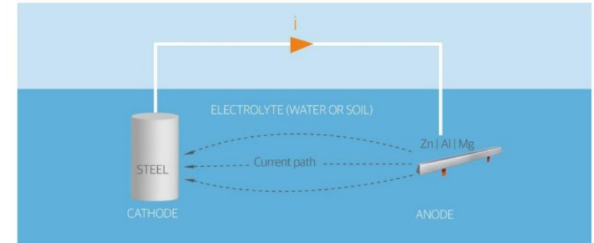
SACRIFICIAL ANODE
